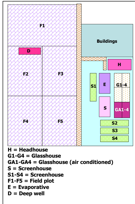
รูปที่ 4 ตัวอย่างแบบแปลนโรงเรือนใหญ่ซึ่งประกอบด้วยโรงเรือนย่อยหลายโรงเรือน
